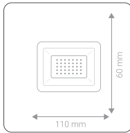
۱۰ وات | 45 mA
