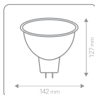
۷ وات | Mr16
